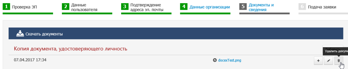
Рис. 3.15 Удаление документа
